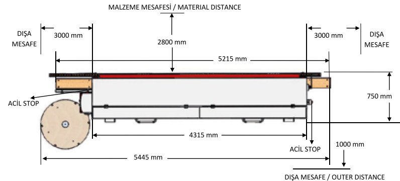
ALT ÜST FREZE BOTTOM & TOP MILLING
